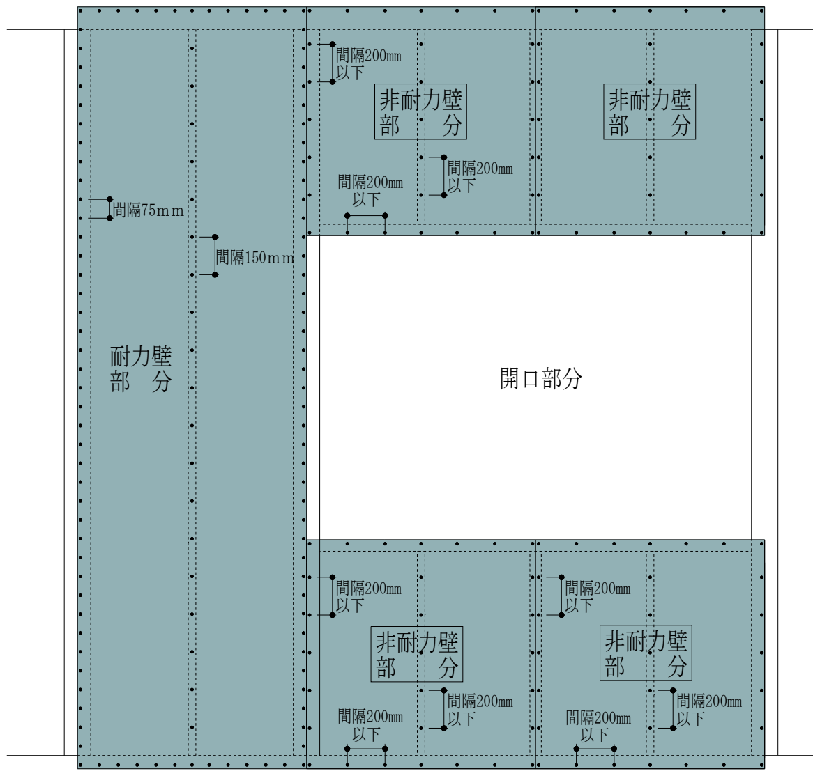
図 21 耐力壁・非耐力壁 納まり図
