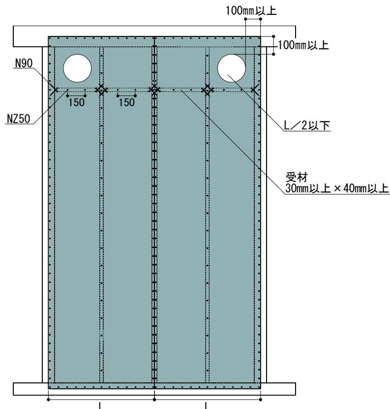
図 19 受材等での補強例*
